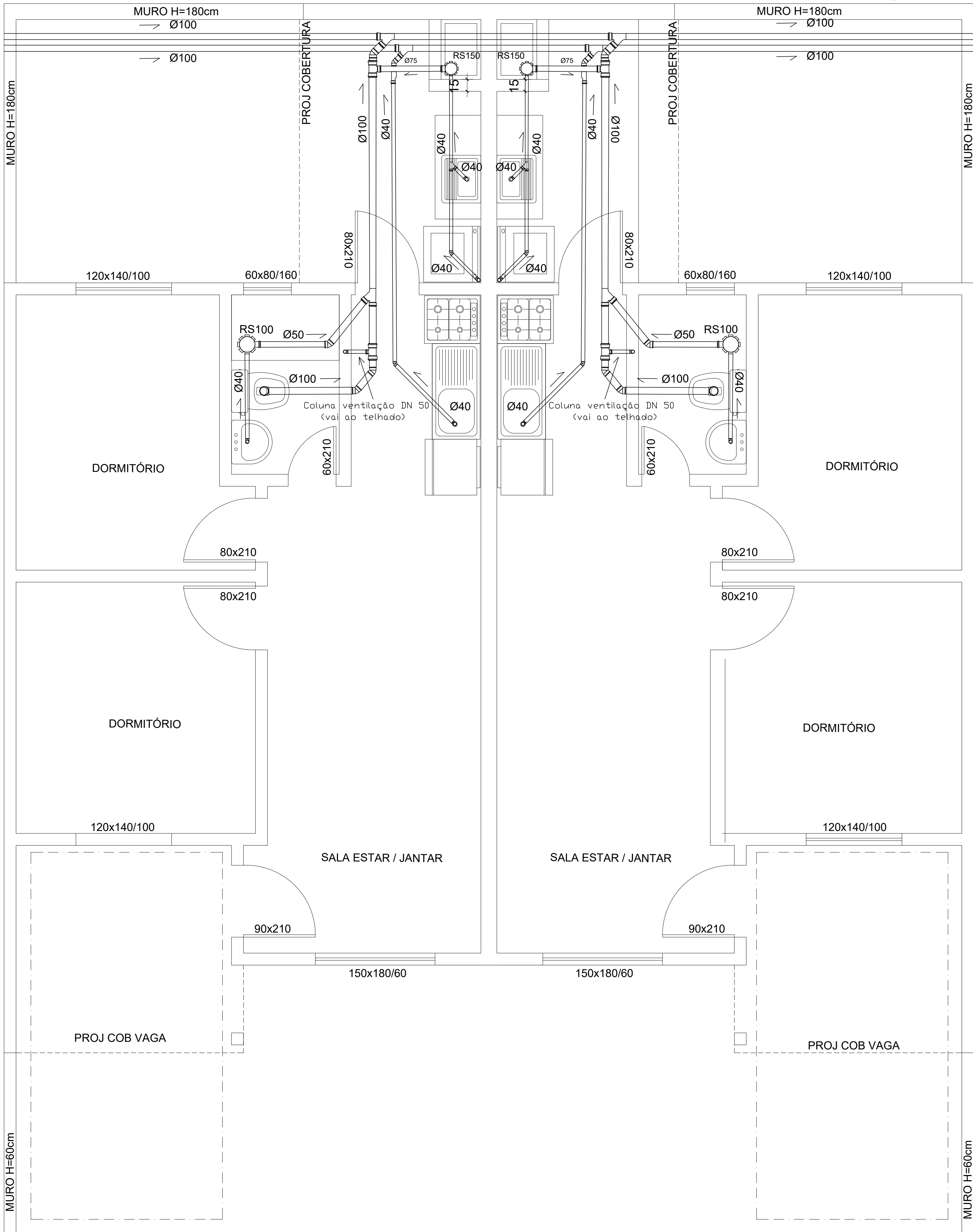
CASAS 02 DORM - DET 02
