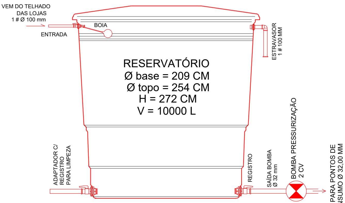
DETALHE 05 ESC.: 1/30
