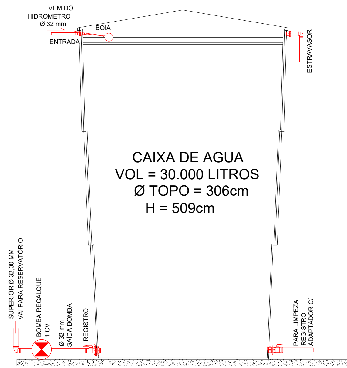
DETALHE 03 ESC.: 1/30
