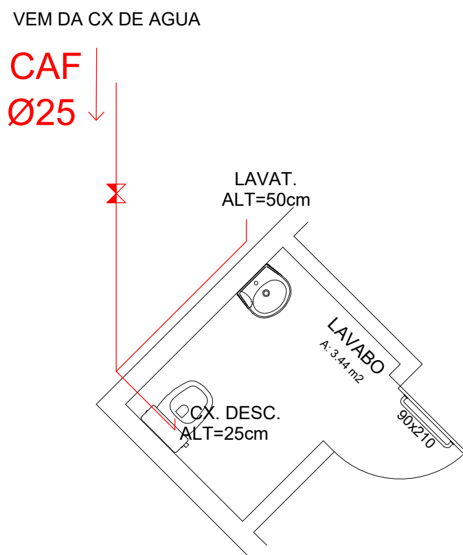
DETALHE 04 ESC.: 1/30
