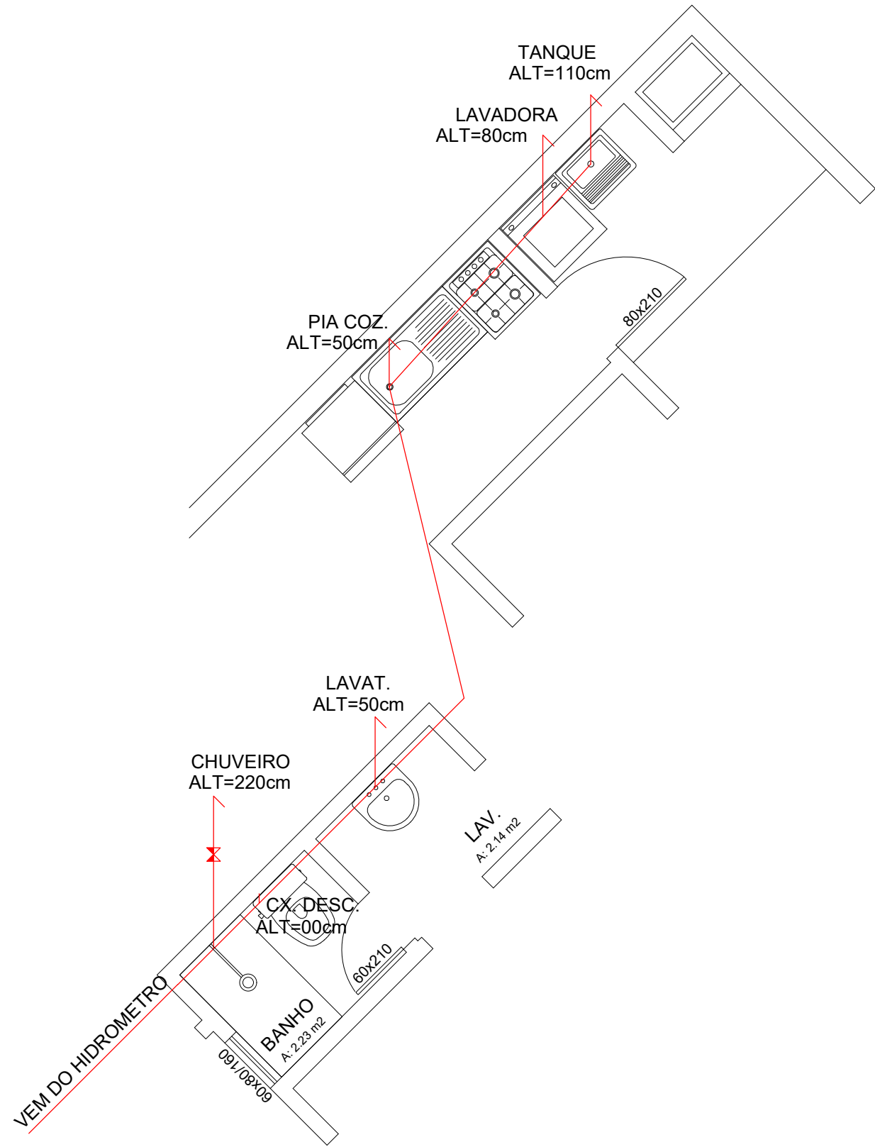
DETALHE 01 ESC.: 1/30
