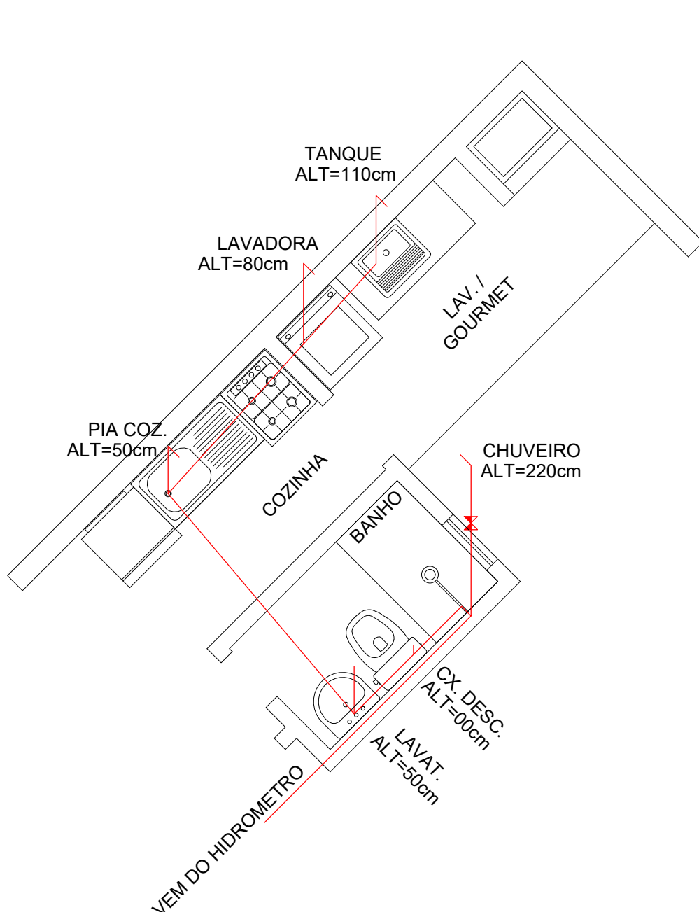
DETALHE 02 ESC.: 1/30
