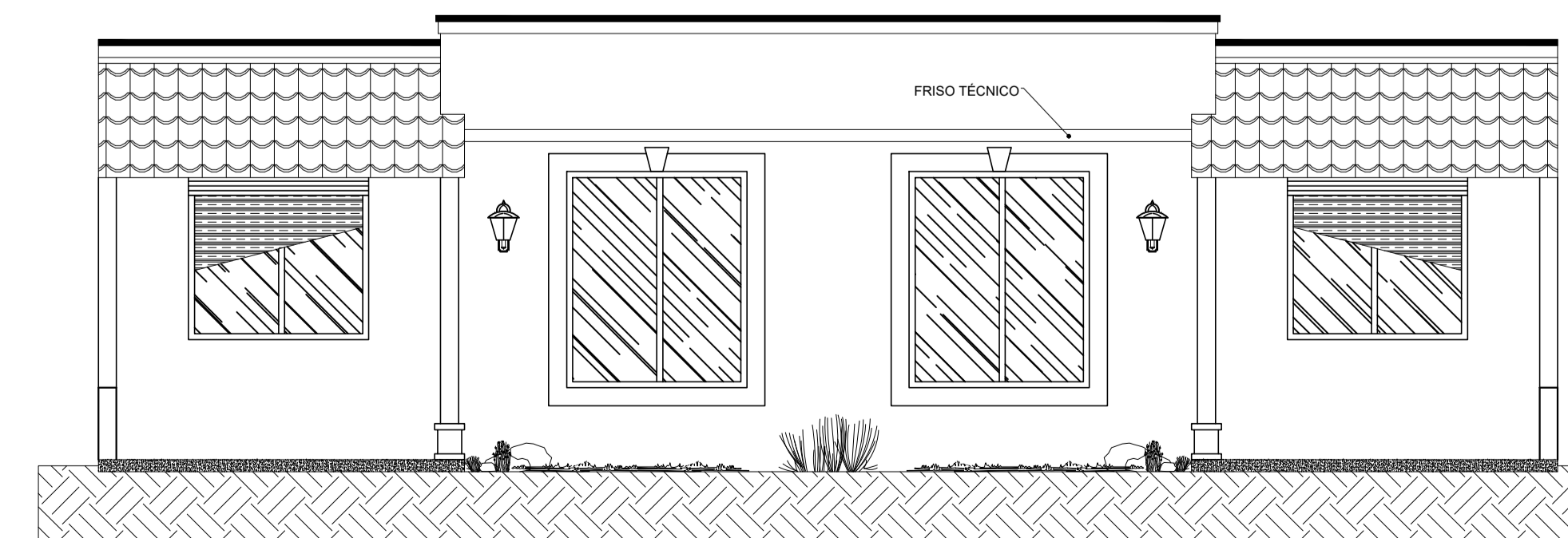
FACHADA CASA 02 DOMRITÓRIOS ESC.: 1/50 (64 REPETIÇÕES)
