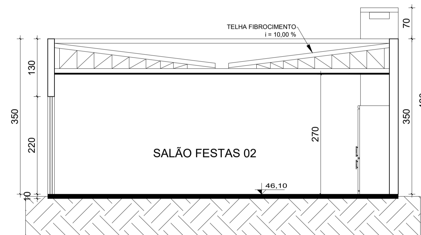
CORTE H-H ESC.: 1/50
