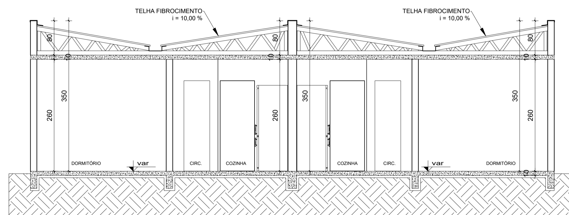
CORTE EE ESC.: 1/50
