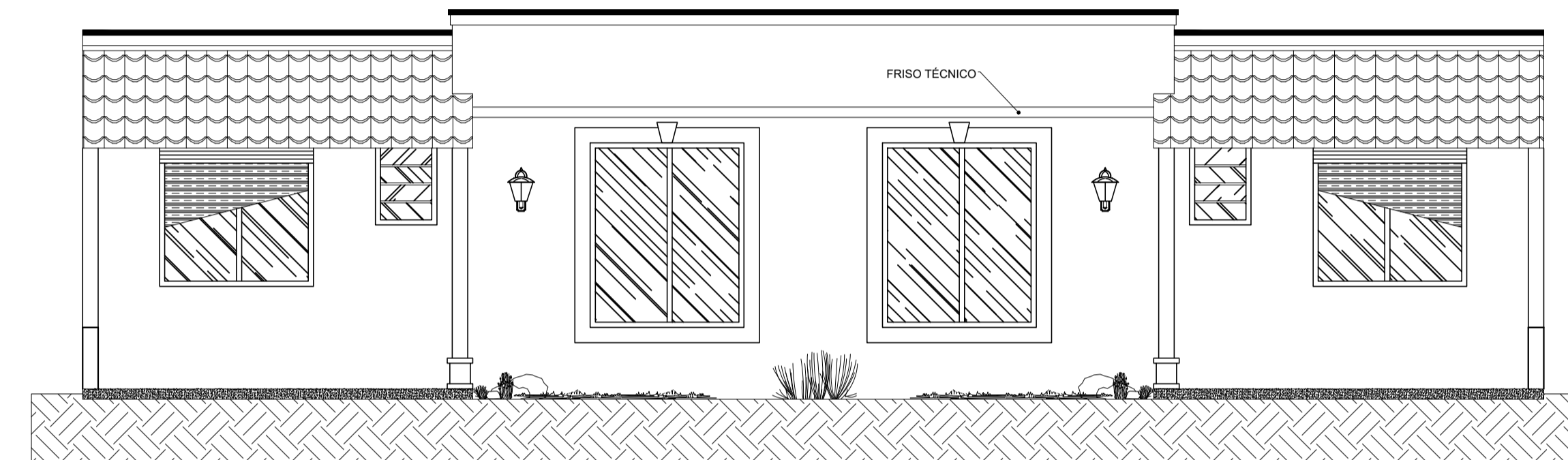
FACHADA CASA 03 DOMRITÓRIOS ESC.: 1/50 (32 REPETIÇÕES)
