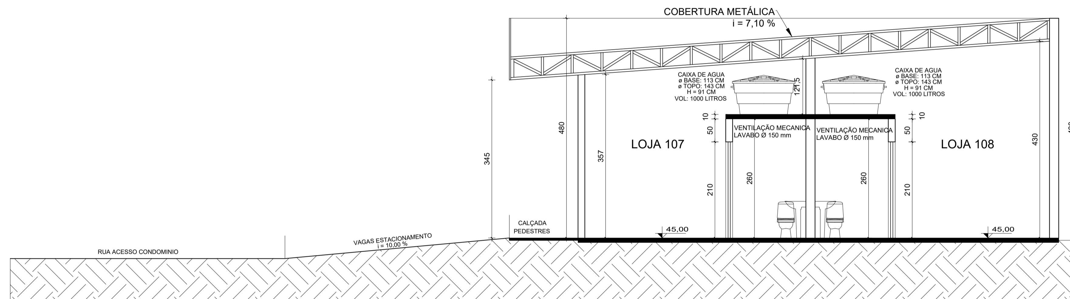
CORTE F-F ESC.: 1/50
