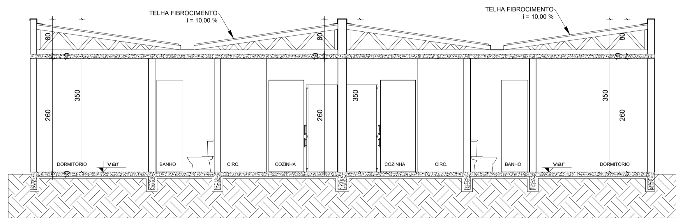
CORTE CC ESC.: 1/50
