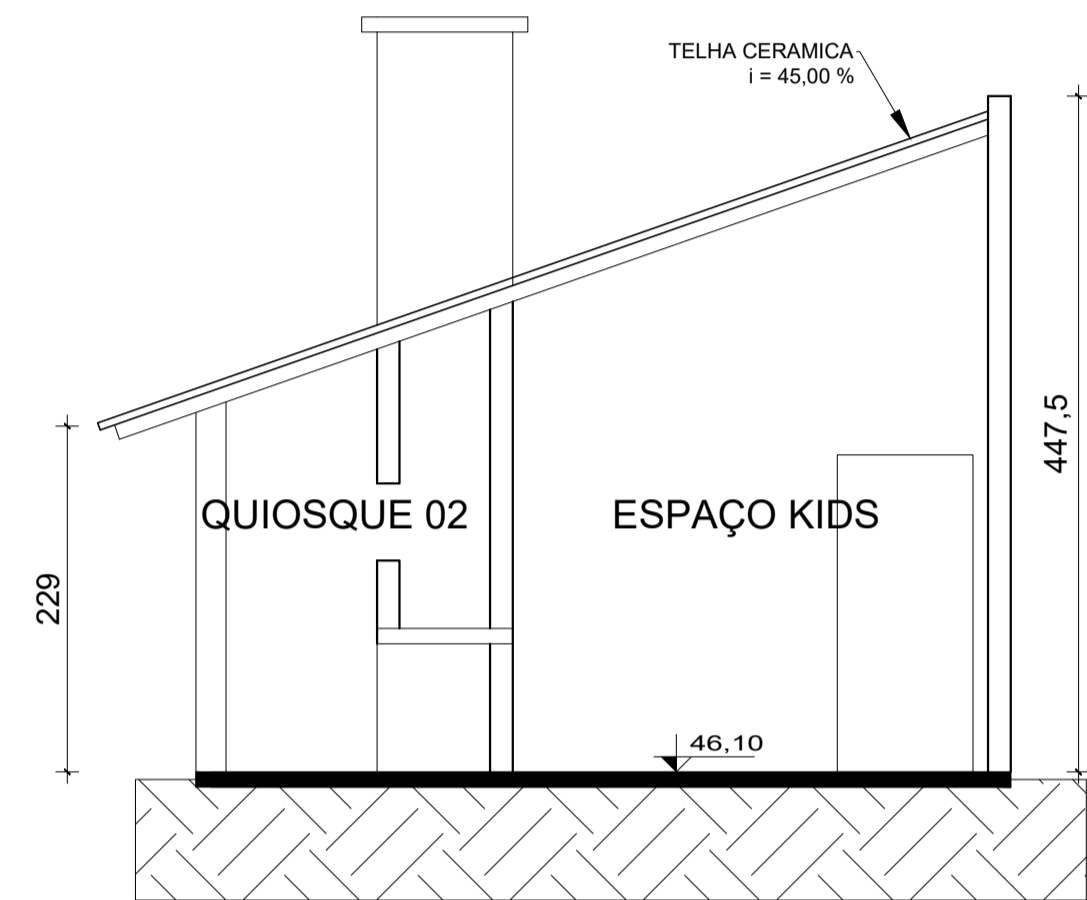
CORTE C-C ESC.: 1/50
