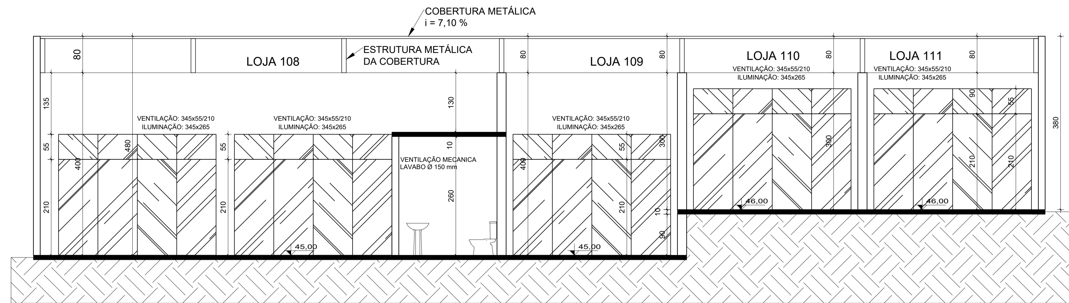
CORTE E-E ESC.: 1/50
