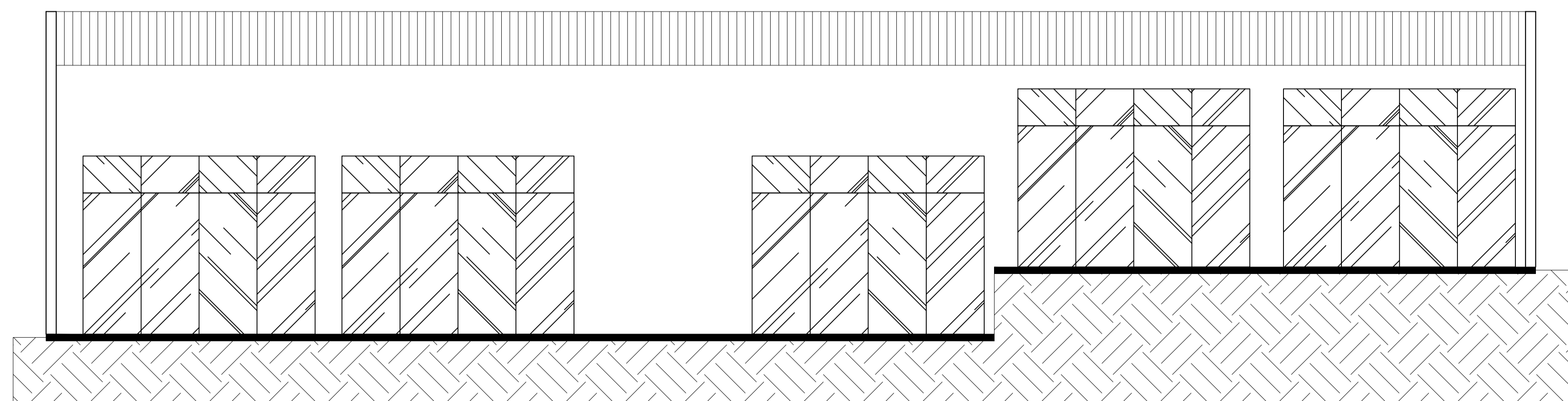
FACHADA FRONTAL LOJAS ESC.: 1/50
