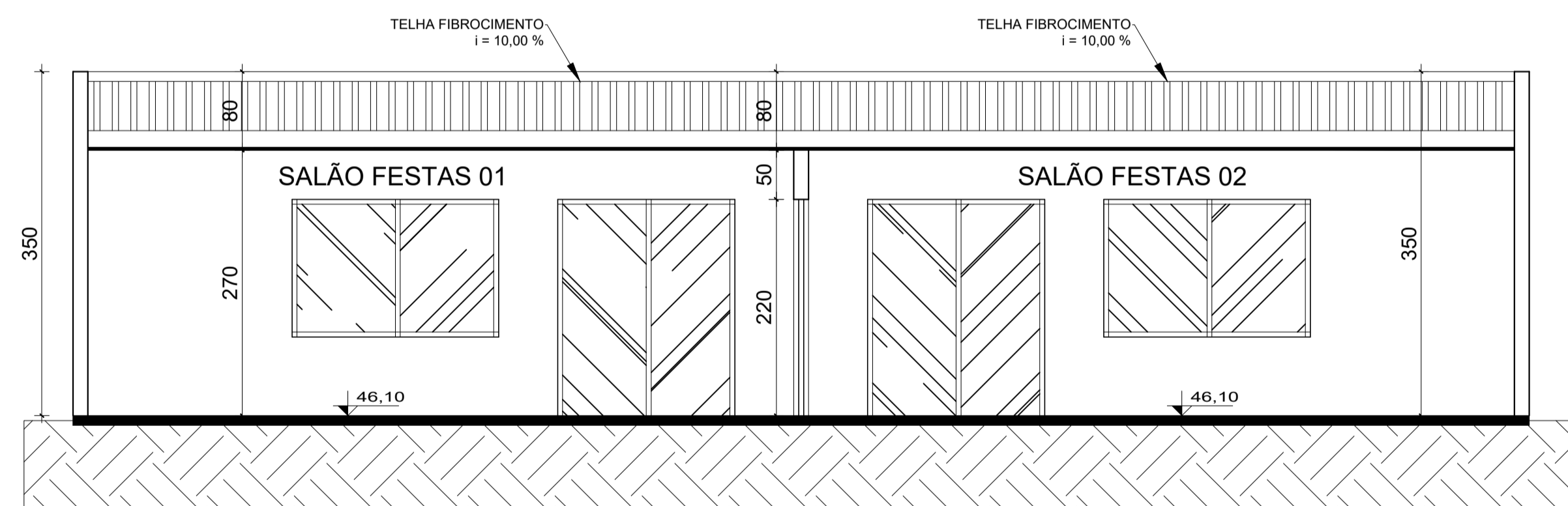
CORTE G-G ESC.: 1/50
