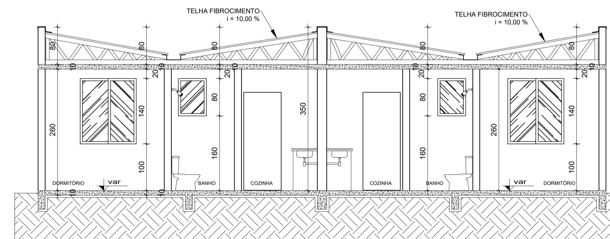
CORTE FF ESC.: 1/50
